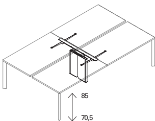
Gamba centrale/salita cavi regolabile in altezza per postazioni doppie
