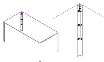
Predisposizione salita cavi nella gamba Solo Nero
