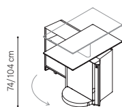
84x50 cm V TDU EL Con elettrificazione CE, UK, US
