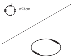
Sportello passacavi tondo e vasca sottopiano per raccolta cavi
