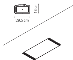
Sportello passacavi rettangolare e vasca sottopiano per raccolta cavi
